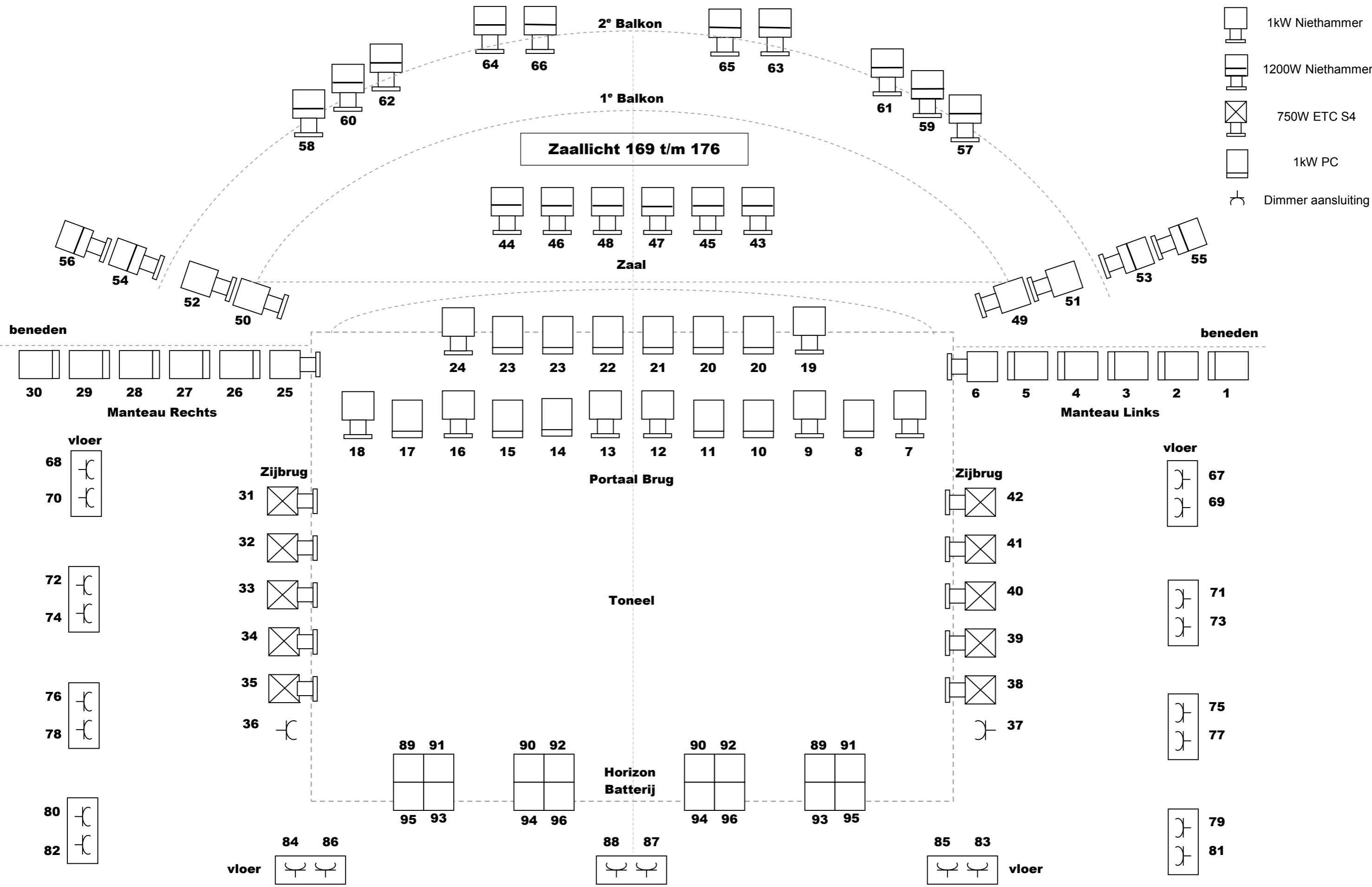
LICHT PLAN LEIDSE SCHOUWBURG
